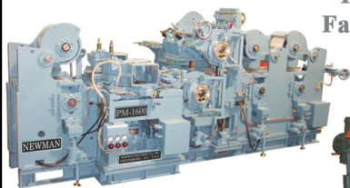
Machimbradora de alta velocidad
